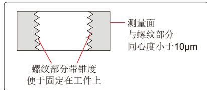
螺纹同心度环规
